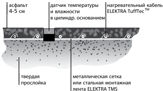
Поперечное сечение дороги или подъездного пути, изготовленного из асфальта
